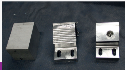
Pièces usinées
